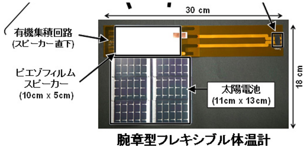
図1 有機集積回路を用いた腕章型フレキシブル体温計
